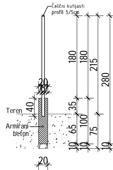
PRESEK 2-2
