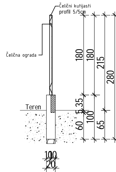
PRESEK 3-3
